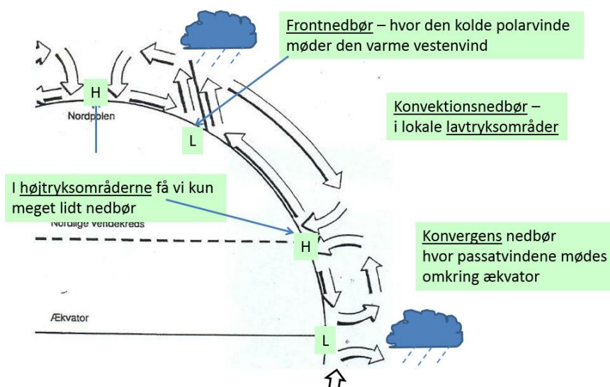
Figur 2 Nedbør finder kun sted under bestemte lufttryk.
