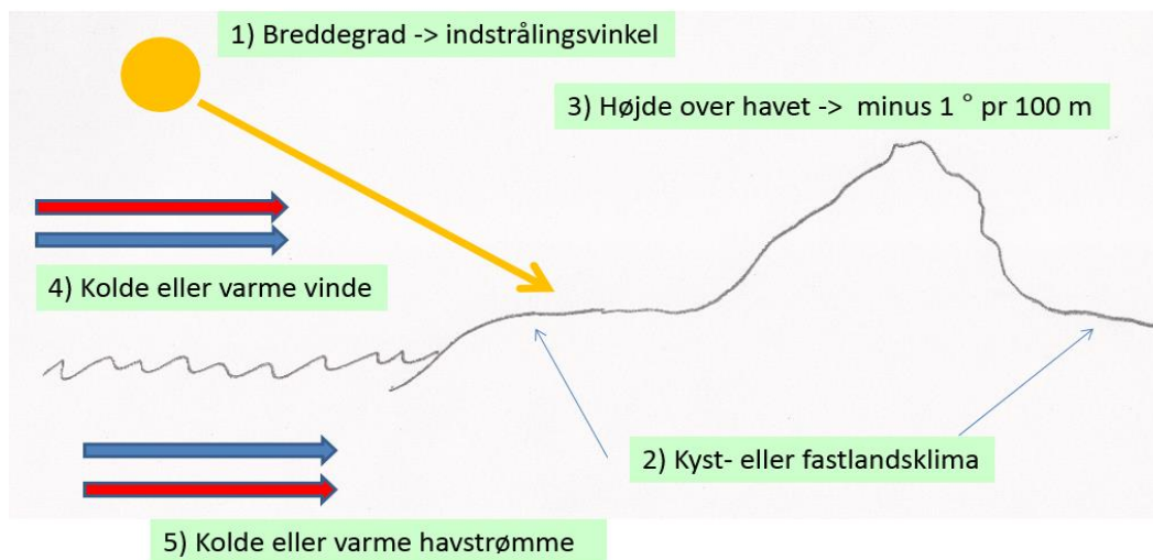
Figur 1 Temperaturforhold er bestemt af en eller flere af disse faktorer
