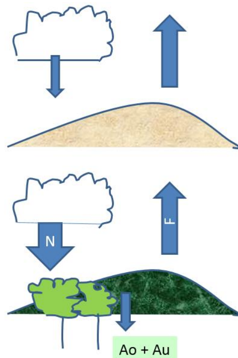
Figur 3 Forholdet mellem nedbør og potentiel fordampning og afstrømning
